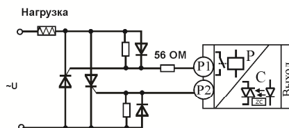
Подключение внешних тиристоров
