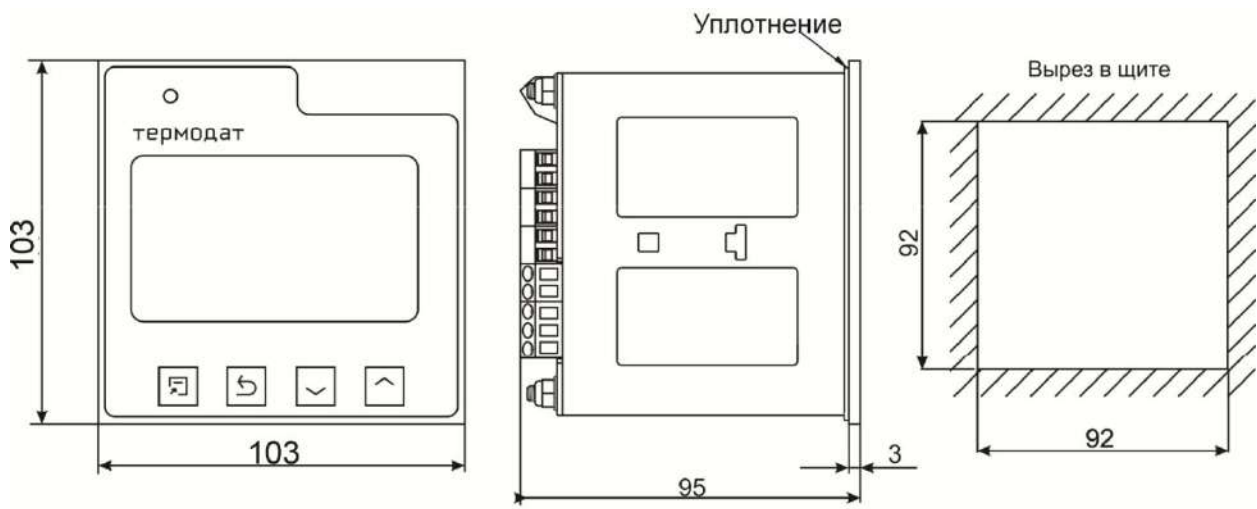
Рисунок 12 – Габаритные размеры прибора Термодат-16К6/...../IP67пп или Термодат-16К6-А7
